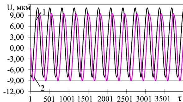
Рисунок 1 – Диаграммы перемещения колодки тормозного механизма
