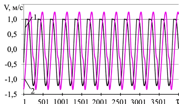
Рисунок 2 – Компоненты скорости перемещений колодки
