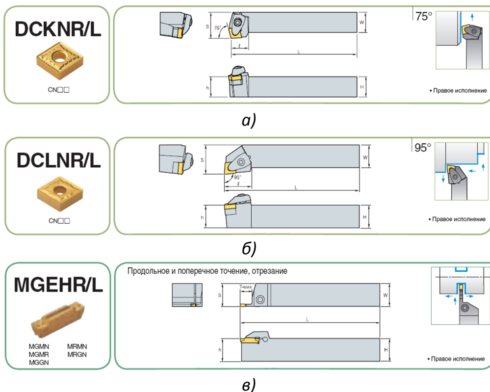
Рис. 3 – Токарные резцы «Korloy» для станка с ЧПУ а) для обработки торцов; б) для наружной обработки; в) для точения канавок
