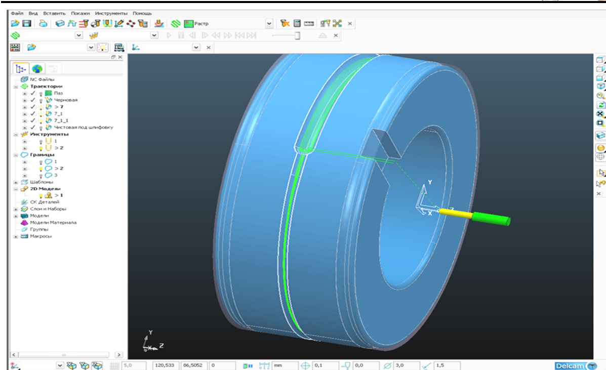
Рис. 7 – Чистовая обработка ручья калибра
