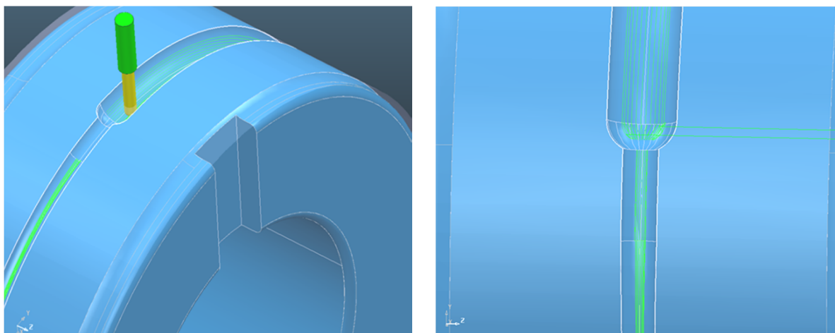
Рис. 8 – Область перехода профиля ручья калибра
