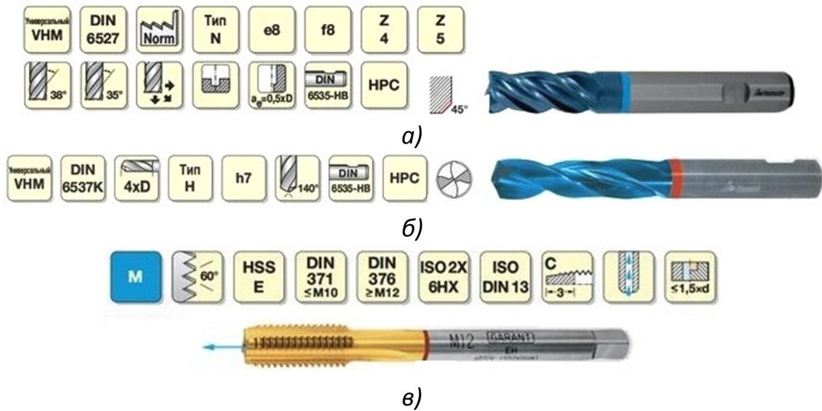
Рис. 4 – Осевой твердосплавный инструмент «Hoffmann Group» а) концевая фреза; б) спиральное сверло; в) метчик с подводом СОЖ
