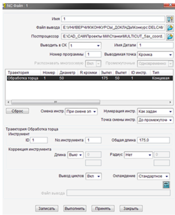
Рис. 12 – Фрагмент УП
