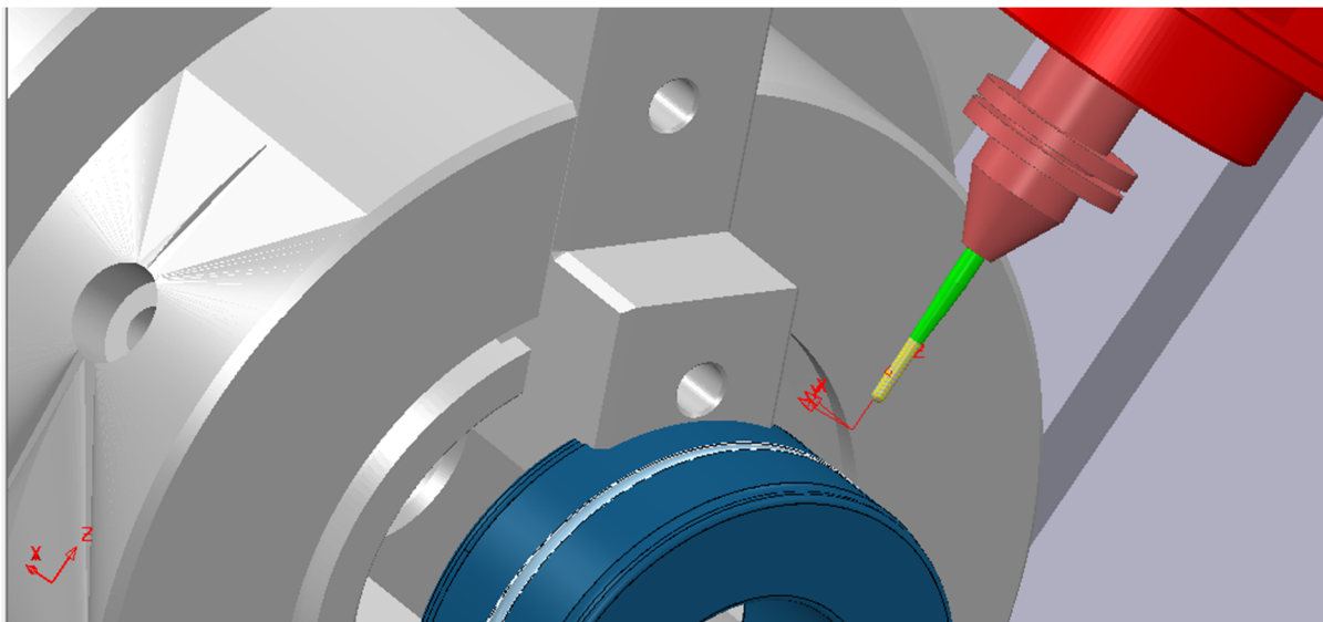
Рис. 11 – Визуализация обработки на станке «OKUMA Mac Turn 250»
