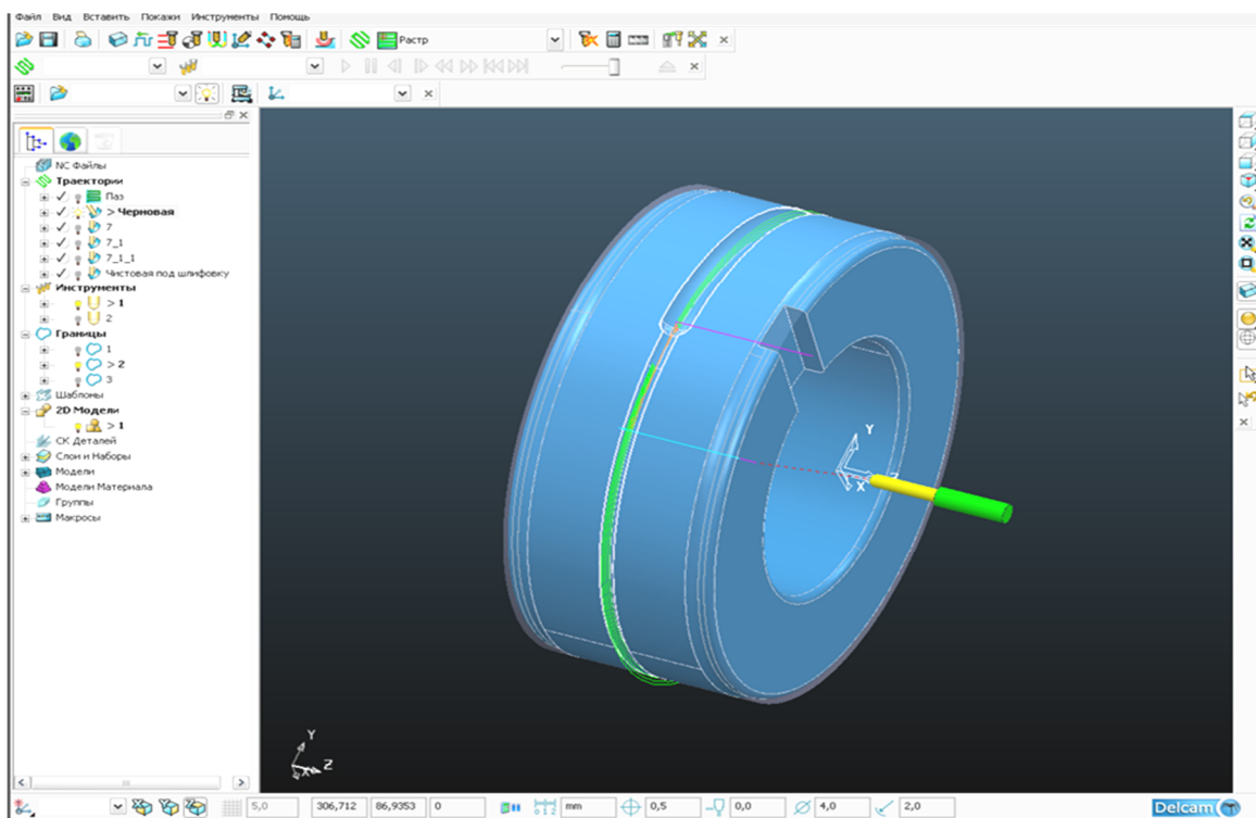
Рис. 6 – Черновая обработка ручья калибра
