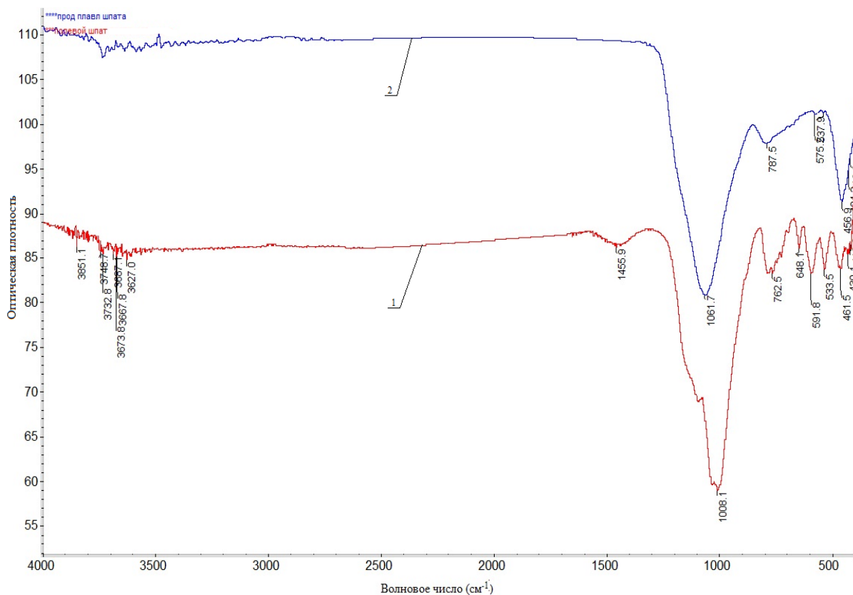
Рисунок 3. ИК–спектры пропускания:
