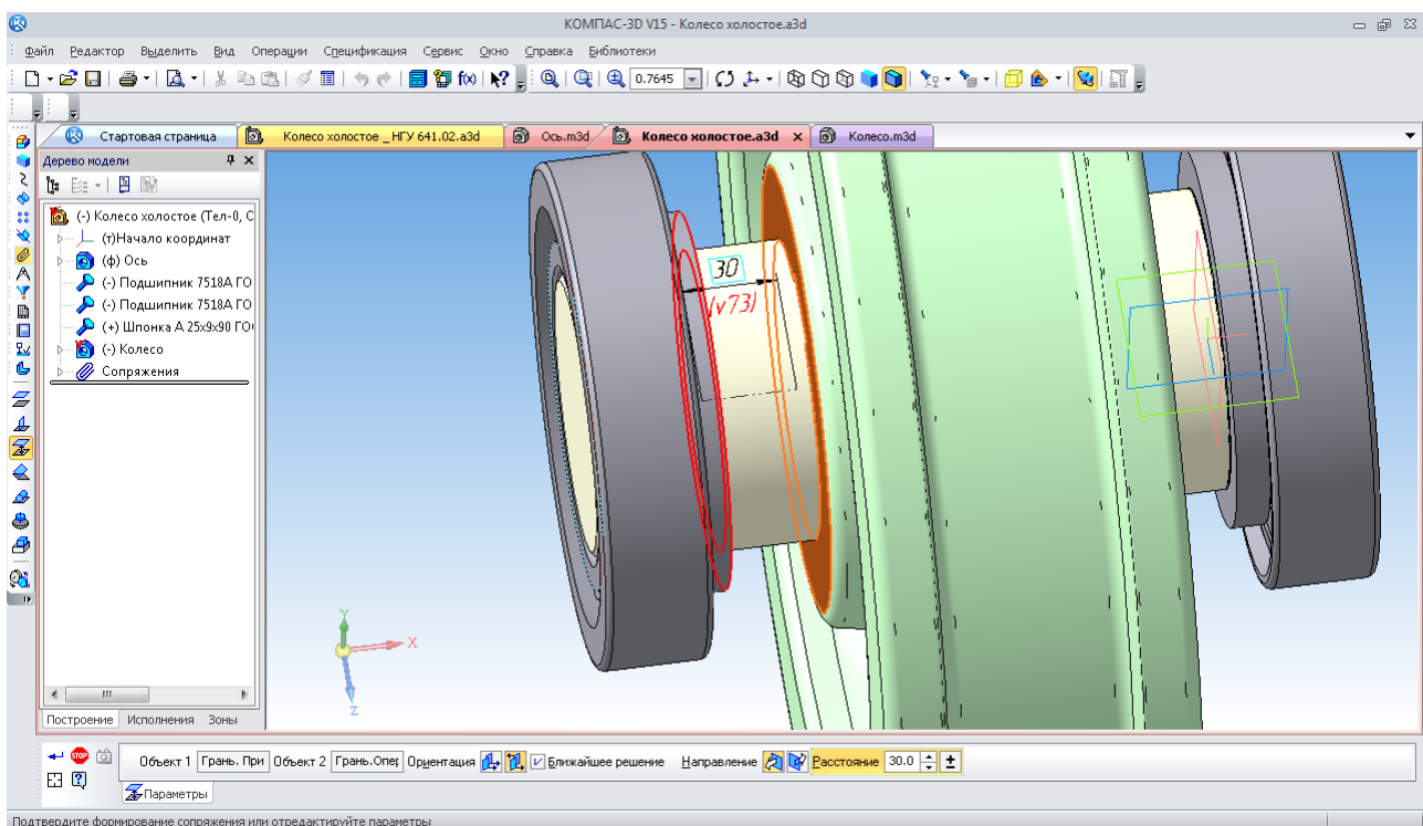
Рис. 162. Накладення сполучення «На расстоянии»
