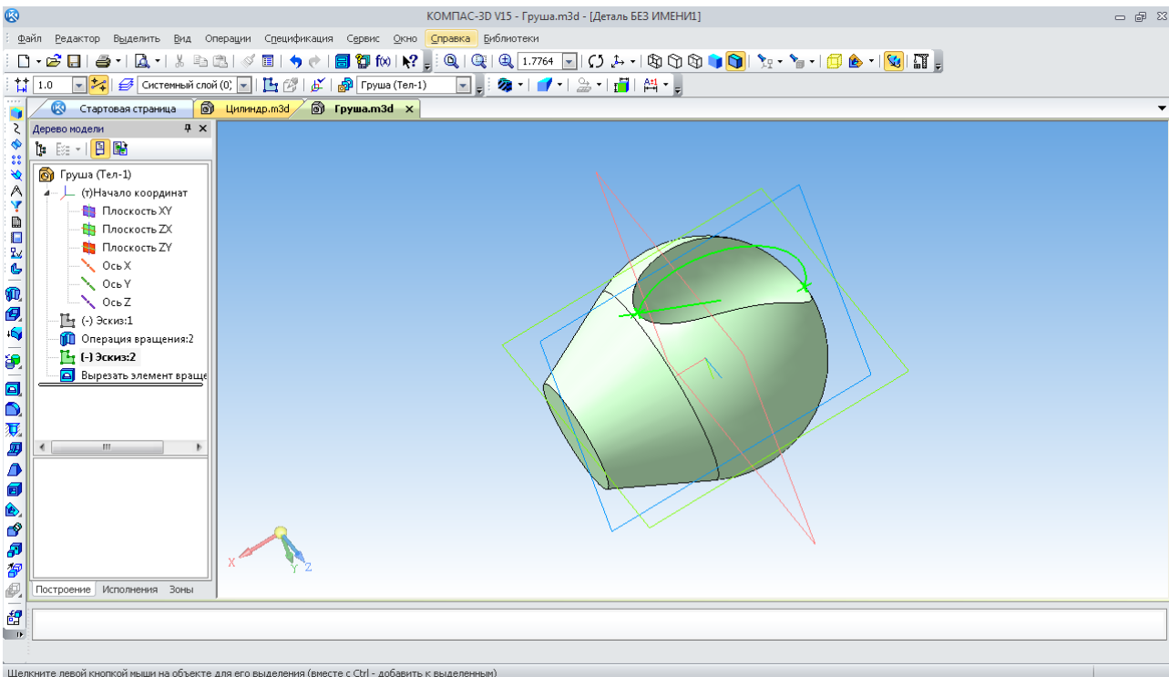
Рис. 90. Модель тіла зі складним фігурним пазом
