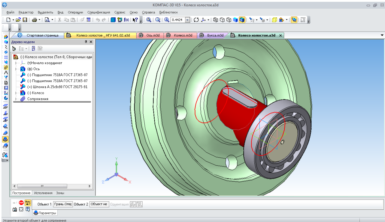
Рис. 159. Накладення сполучення «Соосность»
