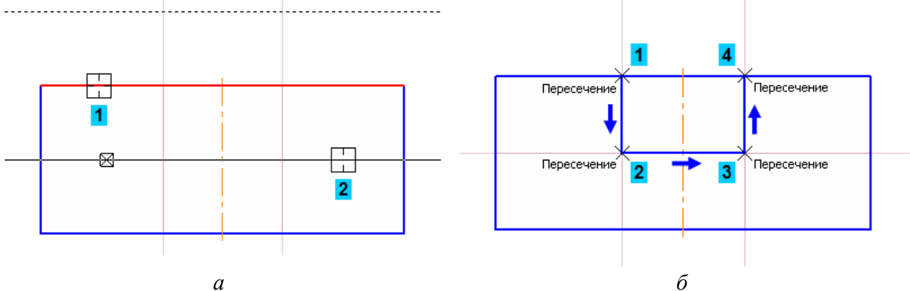
Рис. 46. Побудова паза: а – допоміжною лінією вказують положення паза; б – основні лінії положення паза
