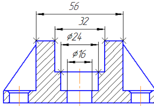
Рис. 62. Проставляння розмірів
