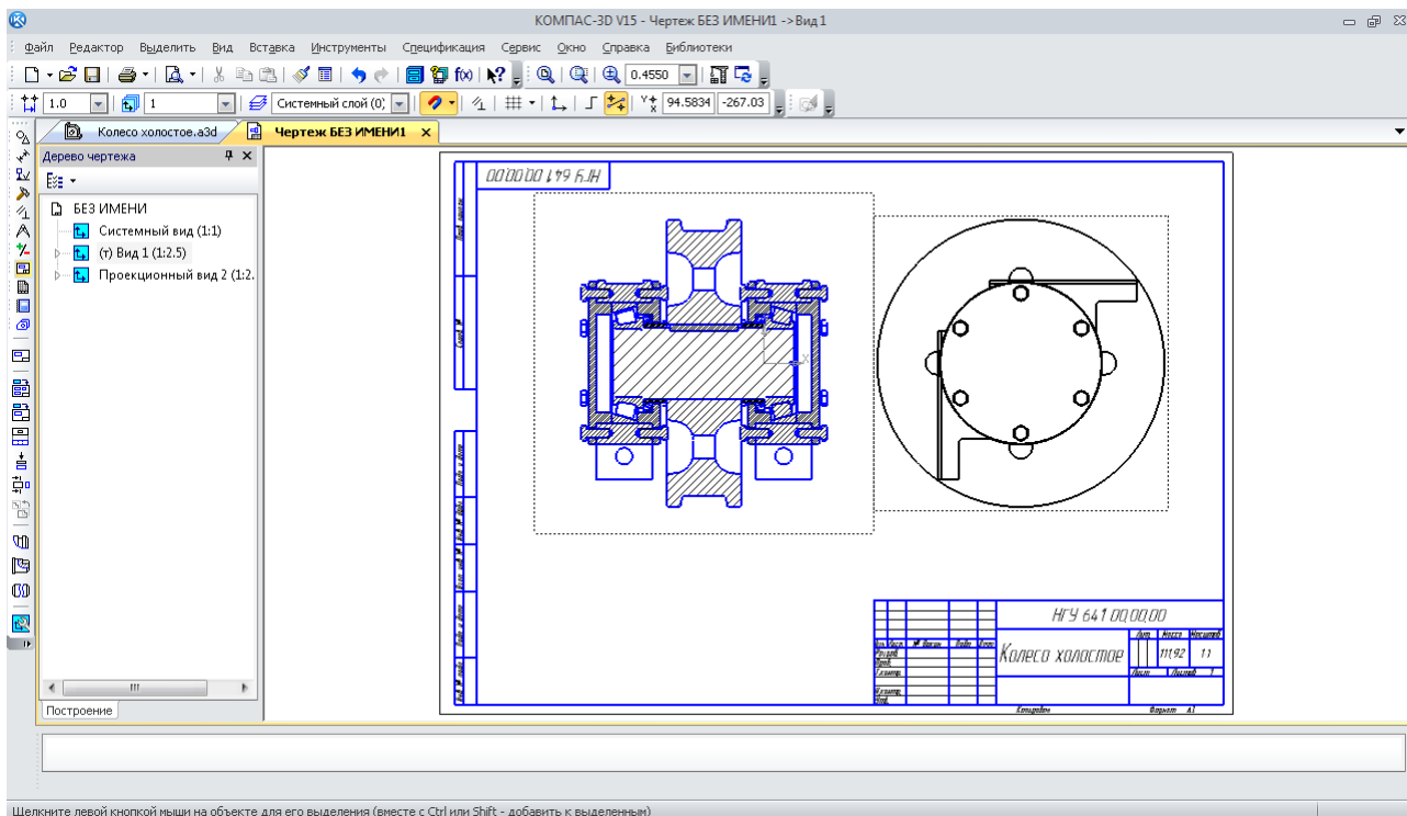
Рис. 199. Достатне число видів на кресленнику
