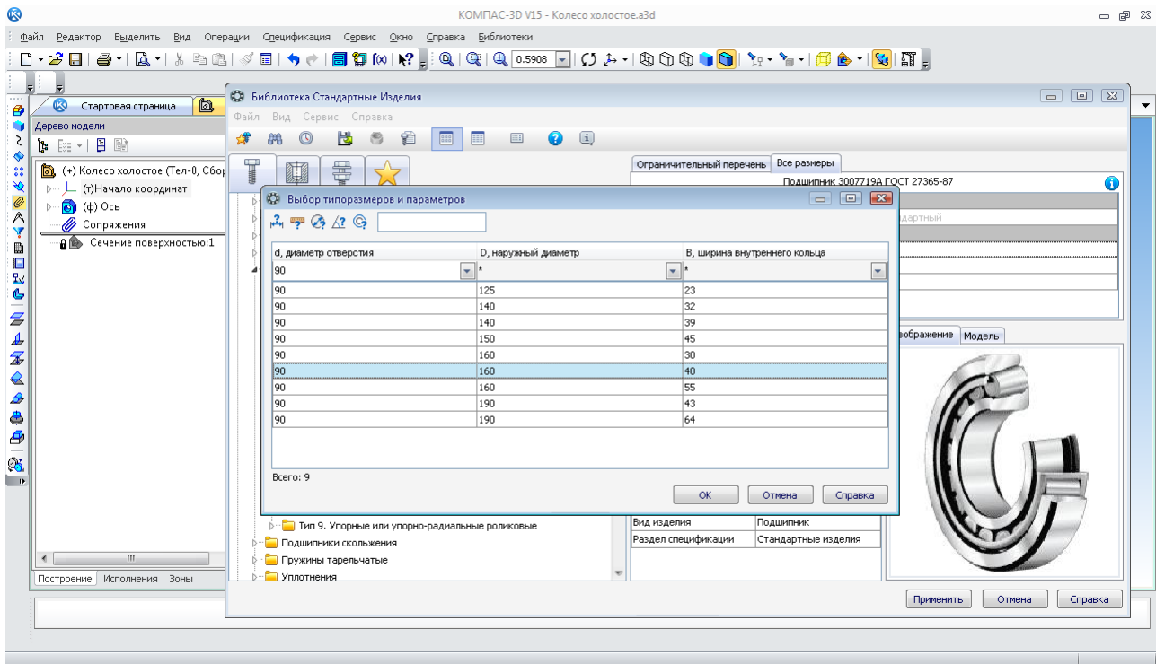
Рис. 149. Вікно для вибору параметрів підшипника
