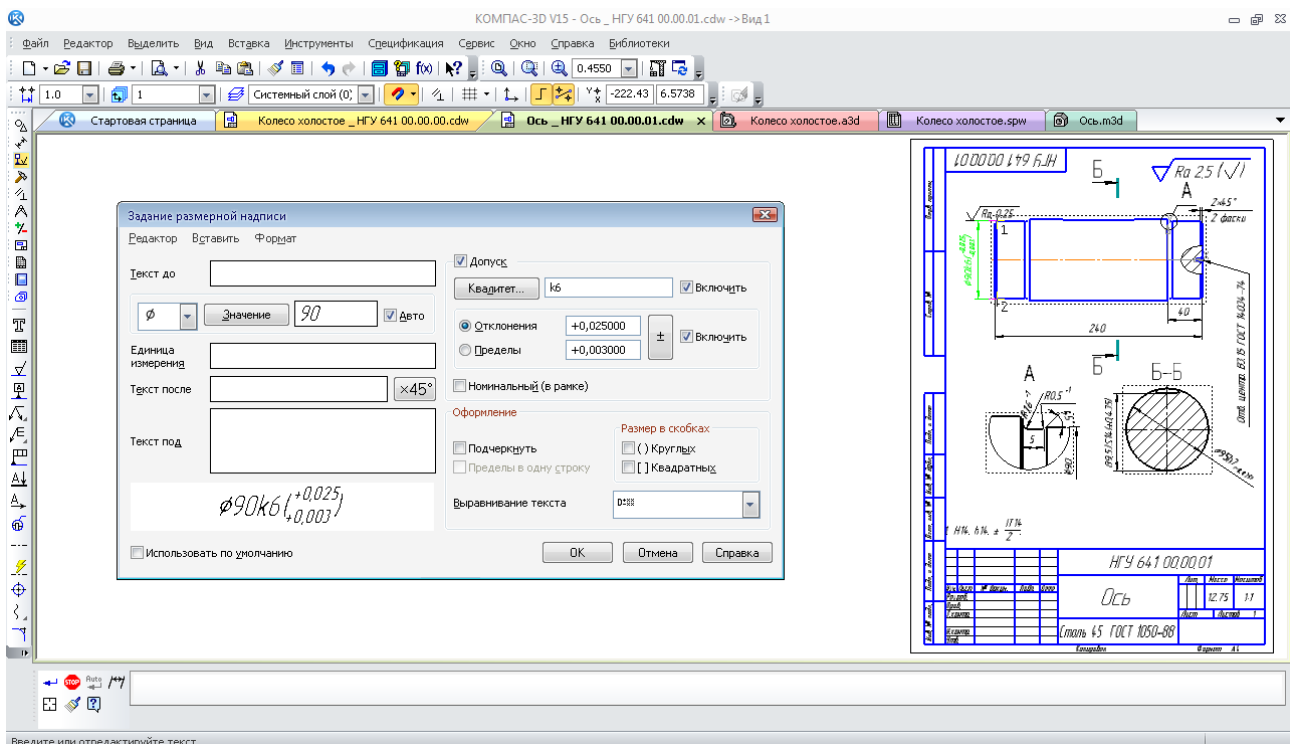
Рис. 214. Розміри з допусками на виготовлення деталі
