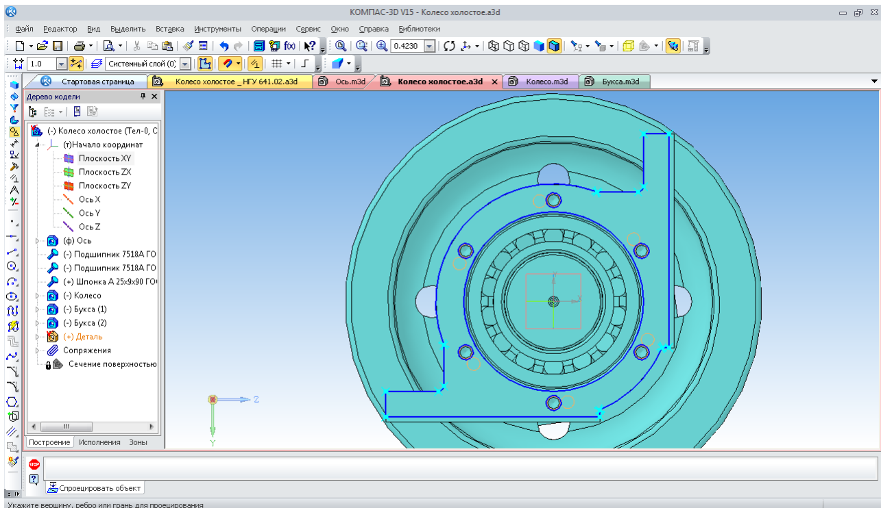
Рис. 166. Використання команди «Спроецировать»
