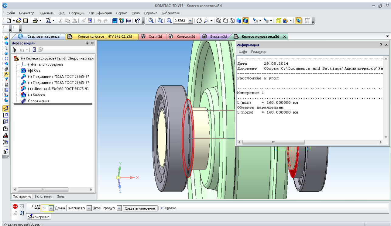
Рис. 161. Вимір відстані між елементами (об'єктами)
