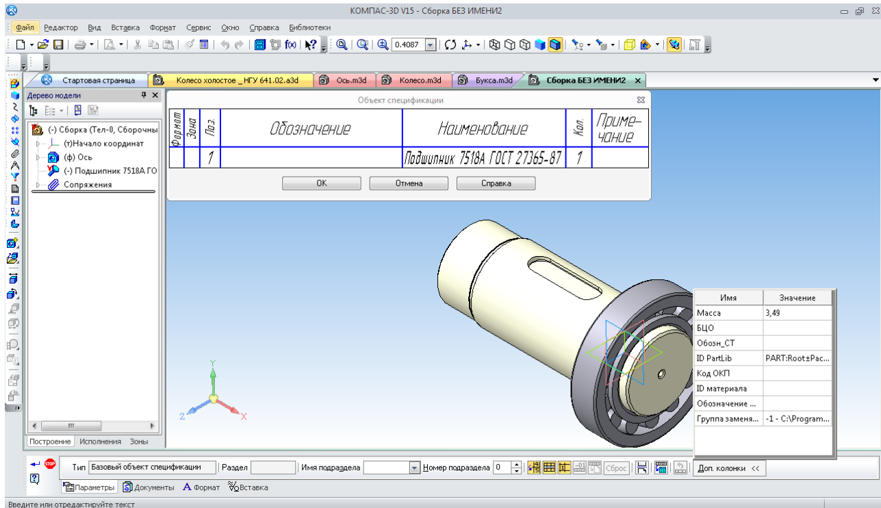
Рис. 151. Підтвердження на створення об'єкта специфікації
