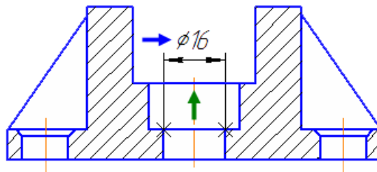
Рис. 60. Нанесення розмірів отвору
