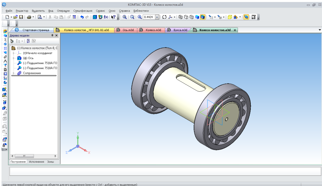
Рис. 152. Розміщення підшипників на деталі «Ось»
