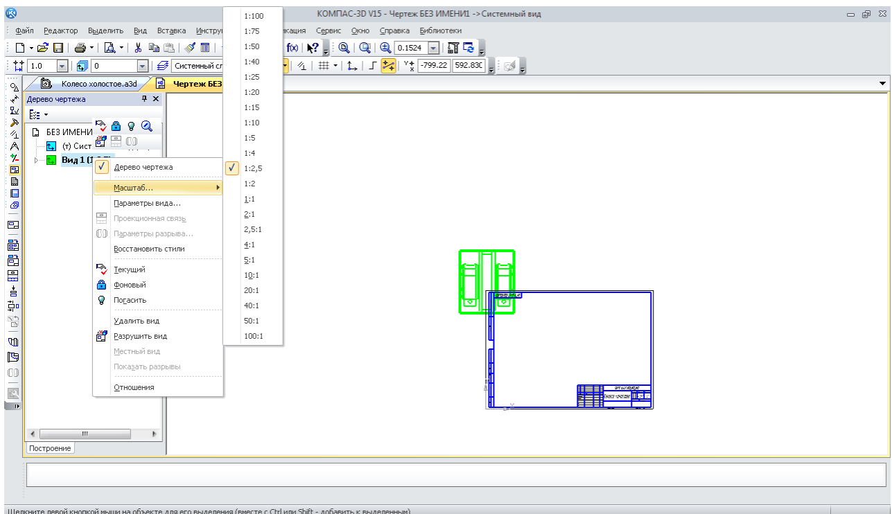
Рис. 198. Налаштування масштабу кресленника
