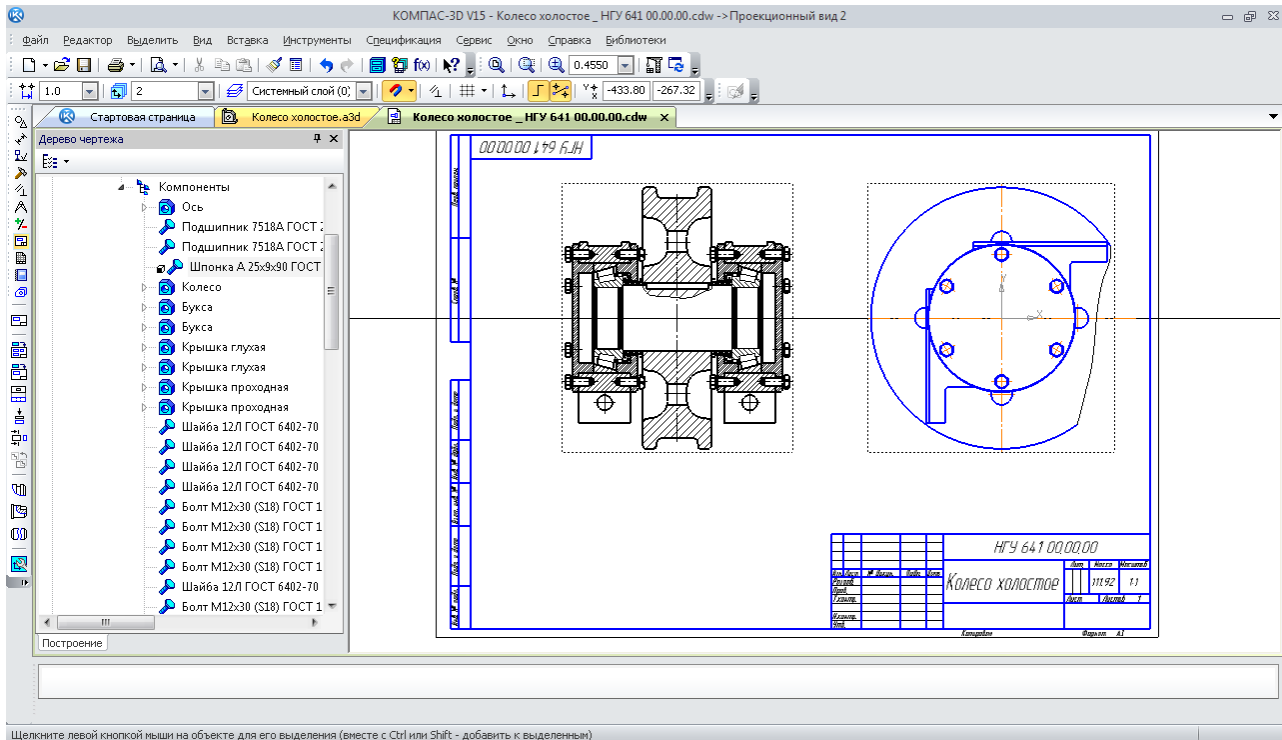
Рис. 209. Місцевий вид
