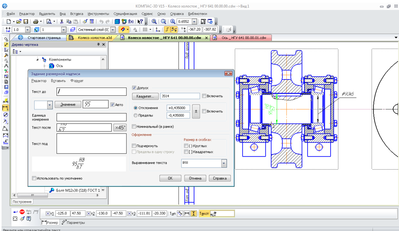
Рис. 211. Нанесення складального розміру з посадкою
