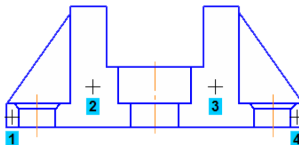
Рис. 51. Переріз деталі перед штрихуванням
