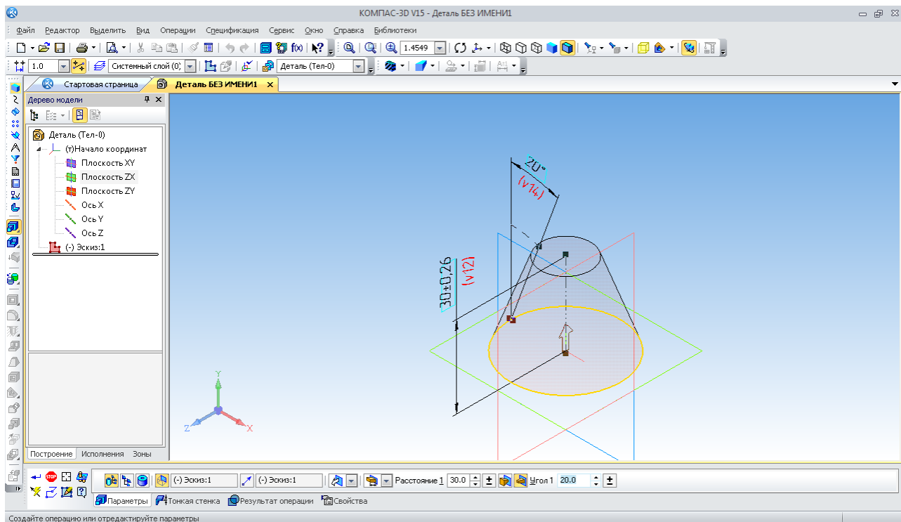
Рис. 75. Побудова усіченого конуса заданням кута
