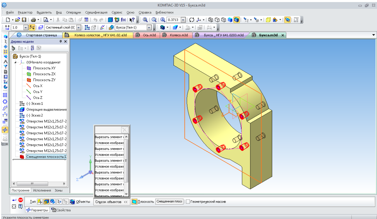
Рис. 143. Побудова дзеркального масиву отворів кріплення
