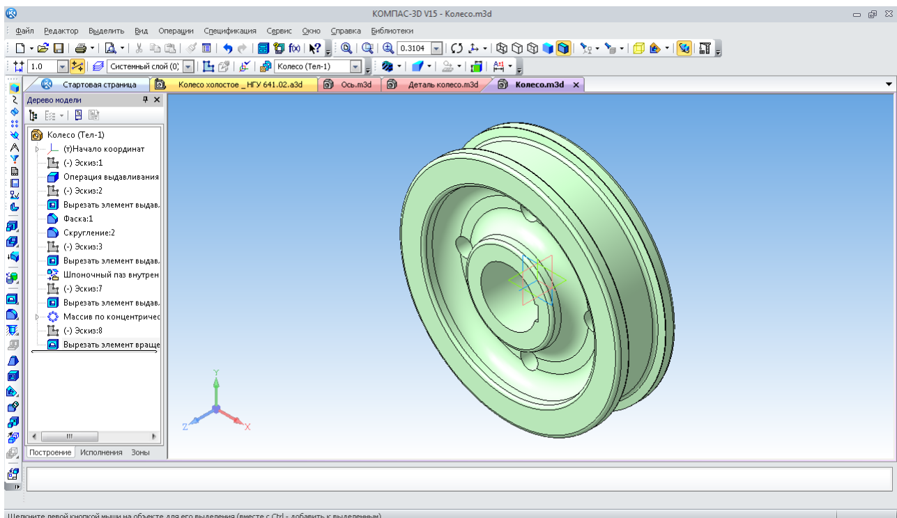
Рис. 134. Тривимірна модель деталі «Колесо»
