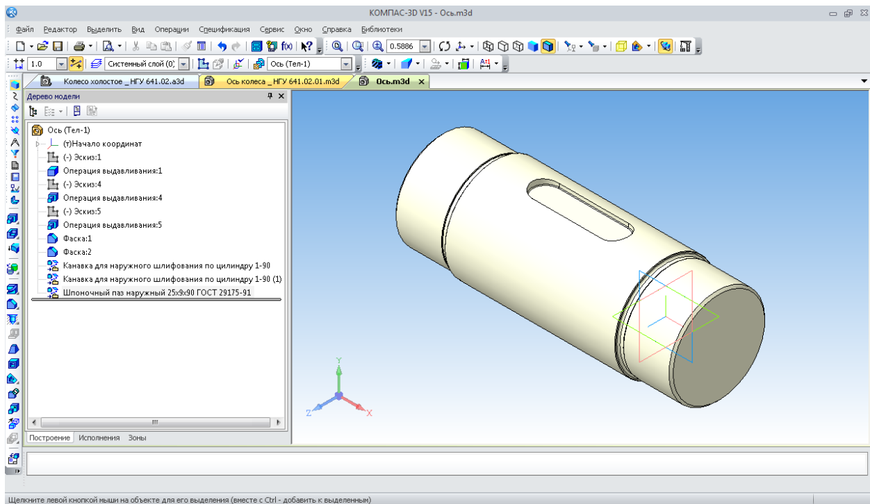
Рис. 120. Шпонковый паз
