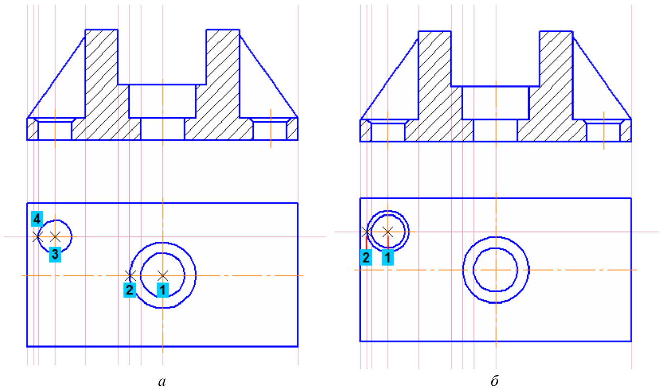
Рис. 55. Побудова кіл: а – отворів; б – фаски
