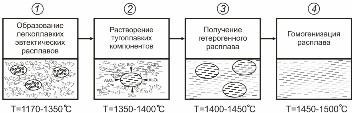
Рисунок 2 – Схема процессов плавления золошлаковых отходов при технических скоростях нагрева
