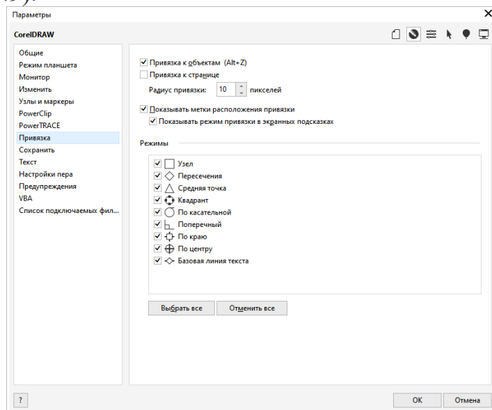
Рис.4.9. Вікно налаштувань об'єктних прив'язок
